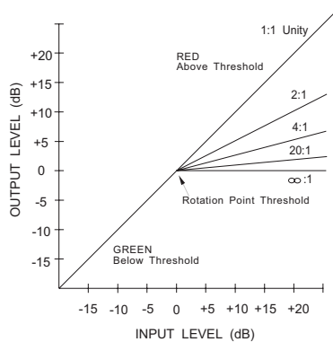
Abb. 1: Hard Knee-Kennlinie und THRESHOLD-LEDs
